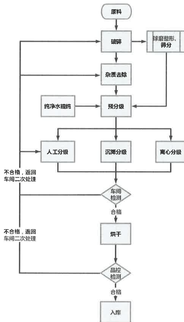
公司工艺流程图
